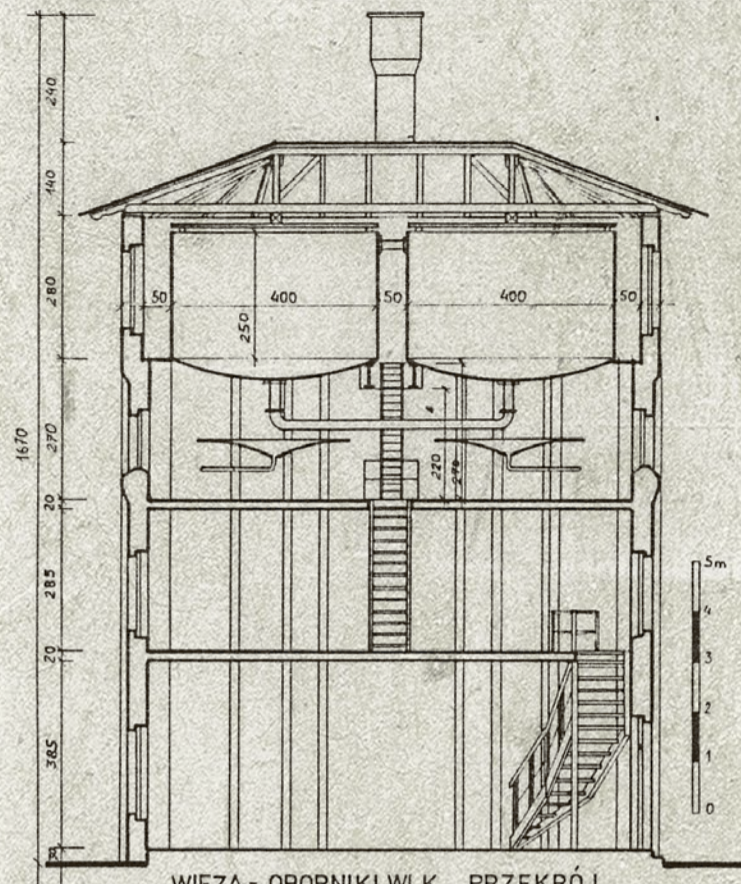
WIEŻA - OBORNIKI WLK. PRZEKRÓJ
